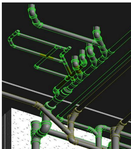
Figura 10: Compatibilização de instalações, arquitetura e estrutura de edificação.
