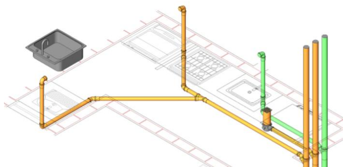
Figura 11: Projeto de esgotamento sanitário confeccionado em plataforma BIM.
